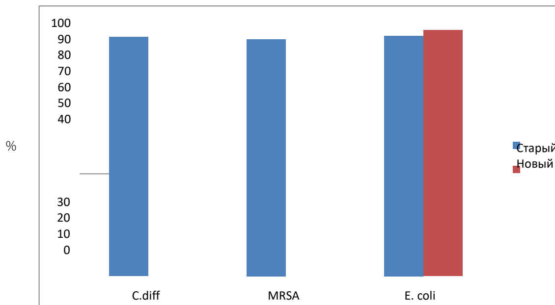
Схема 1б. Результаты очистки, представленные в виде процентного сокращения для микрофибровых салфеток Vikan старого и нового образца после 75 стирок
